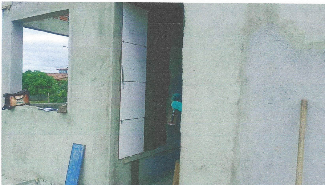
Foto 19 – REVESTIMENTO CERÂMICO PARA PAREDES INTERNAS COM PLACAS TIPO ESMALTADA EXTRA DE DIMENSÕES 33X45 CM APLICADAS EM AMBIENTES DE ÁREA MAIOR QUE 5 M 2 NA ALTURA INTEIRA DAS PAREDES. AF_06/2014
