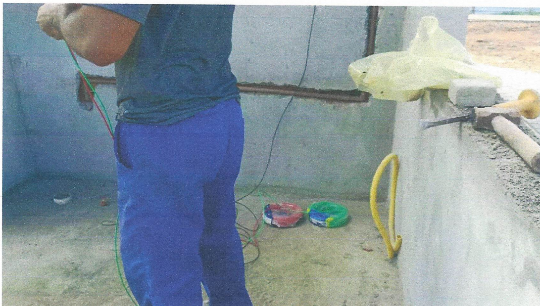
Foto 35 – CABO DE COBRE FLEXÍVEL ISOLADO, 2,5 MM 2 , ANTI-CHAMA 450/750 V, PARA CIRCUITOS TERMINAIS - FORNECIMENTO E INSTALAÇÃO. AF_12/2015.
