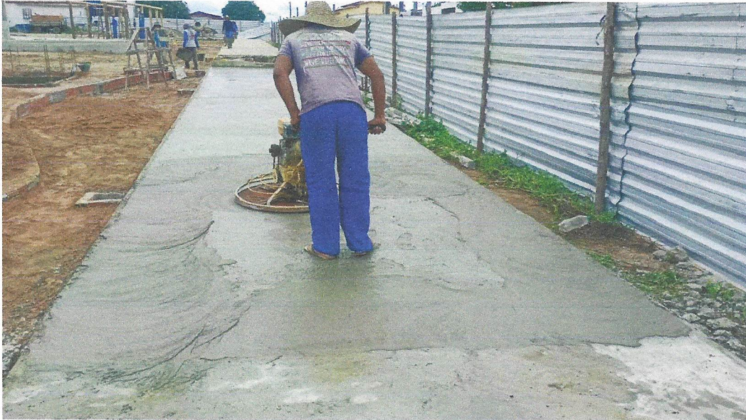
Foto 31 – EXECUÇÃO DE PASSEIO (CALÇADA) OU PISO DE CONCRETO COM CONCRETO MOLDADO IN LOCO, FEITO EM OBRA, ACABAMENTO CONVENCIONAL, ESPESSURA 6 CM, ARMADO. AF_07/2016
